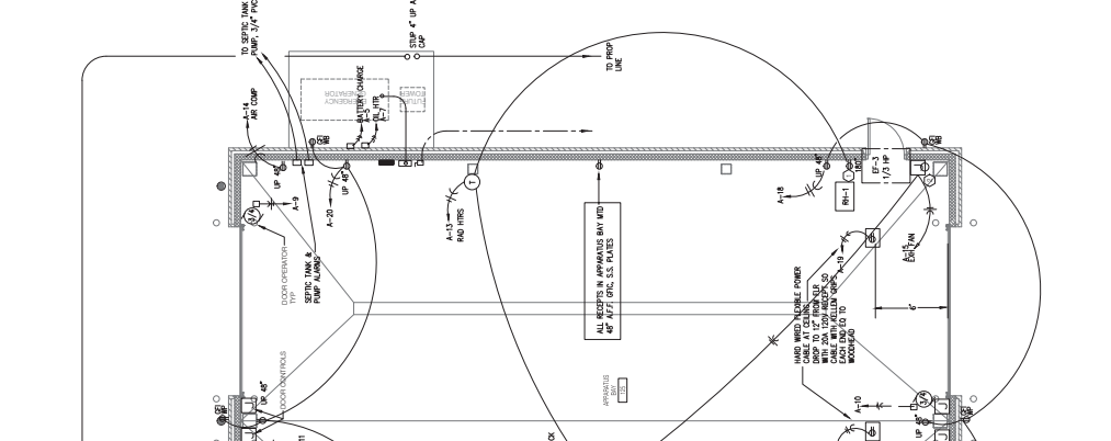
ELECTRICAL ONE-LINE 2 N.T.S. E1.0
